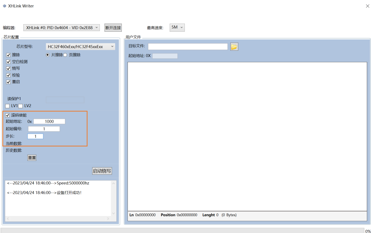
图 4-5 滚码设置
